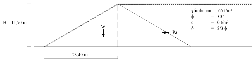
Gambar 7. Sketsa lereng dan tekanan tanah aktif yang bekerja
