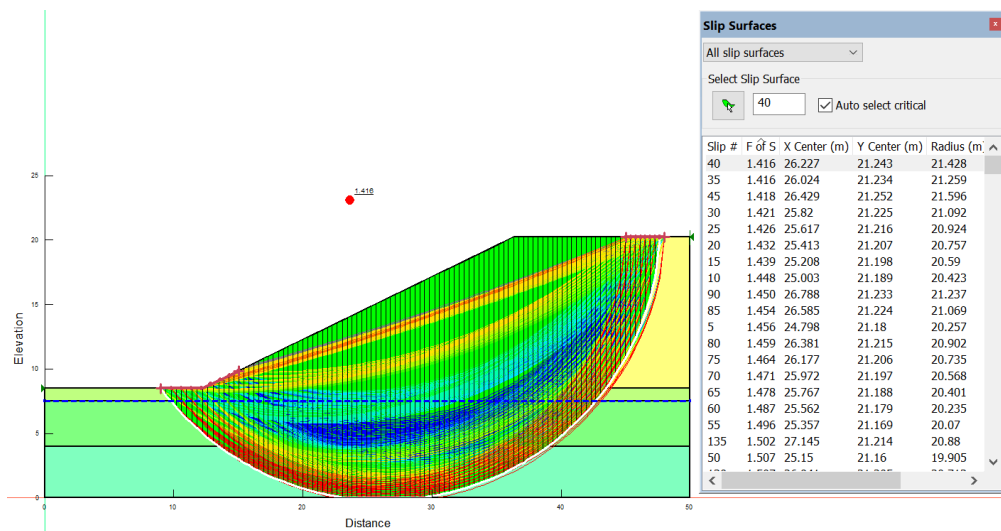
b. Hasil analisis 2 kelongsoran pada lereng timbunan tanpa perkuatan
