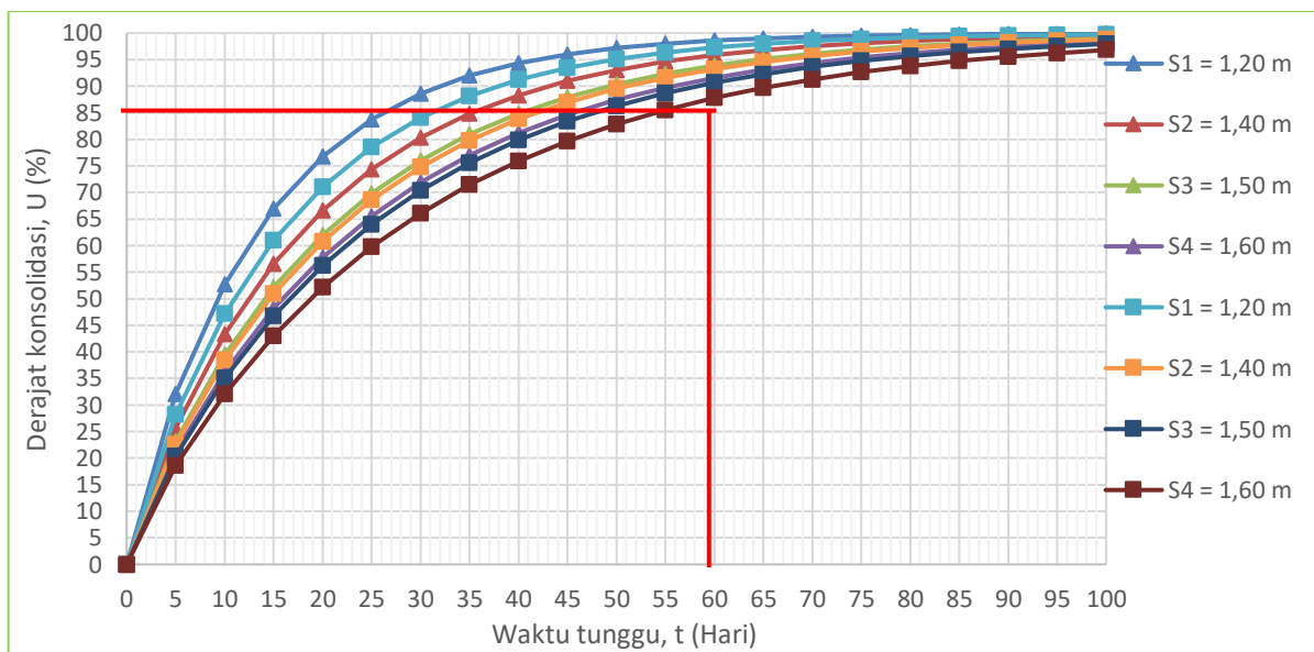
Gambar 6. Grafik hubungan antara derajat konsolidasi (U) dan waktu tunggu (t) pola pemasangan segiempat dan segitiga
