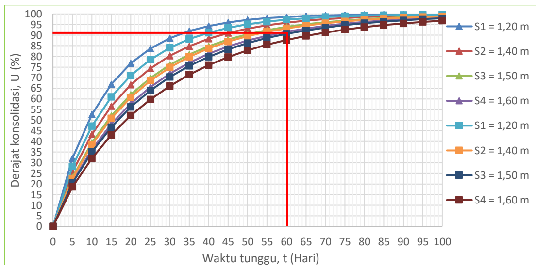
Gambar 12. Grafik hubungan antara derajat konsolidasi (U) dan waktu tunggu (t) pola pemasangan segiempat dan segitiga
