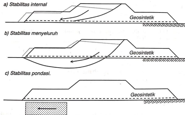
Gambar 2. Mekanisme keruntuhan timbunan bertulang pada tanah lunak (Jewell, 1988) Sumber: Hardiyatmo (2013)
