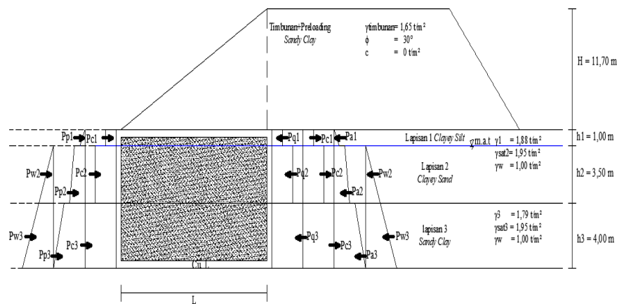
Gambar 8. Sketsa lereng dan tekanan tanah aktif dan pasif yang bekerja
