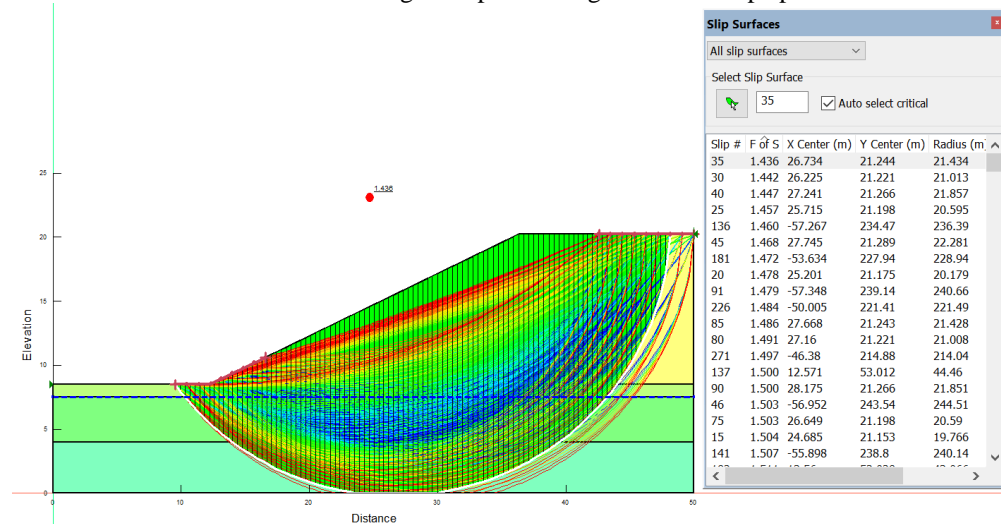
c. Hasil analisis 3 kelongsoran pada lereng timbunan tanpa perkuatan
