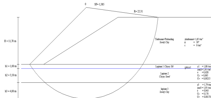
Gambar 11. Bidang longsor lereng tanpa perkuatan
