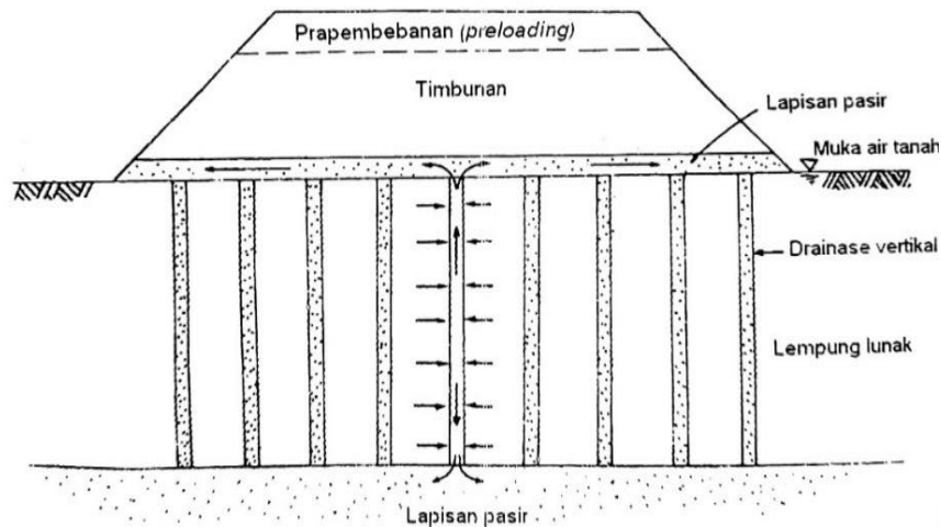
Gambar 1. Skema struktur drainase vertikal
