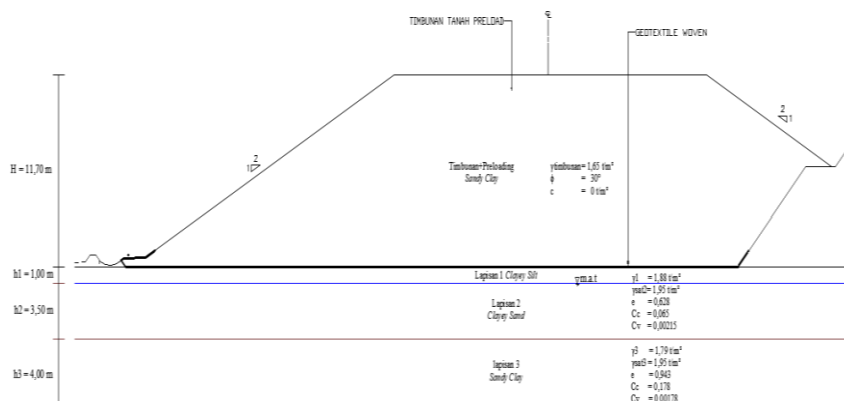
Gambar 5. Permodelan lapisan tanah
