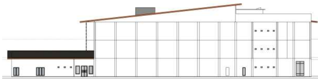
Gambar 15. Tampak Belakang
