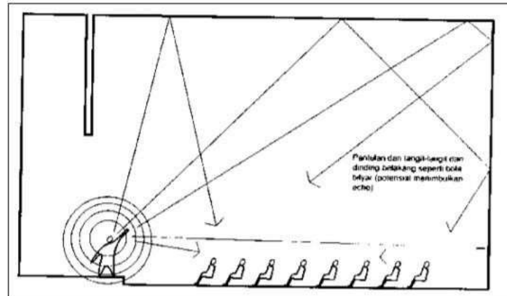
Gambar 6. Pantulan Bunyi Pada Langit-Langit Datar
