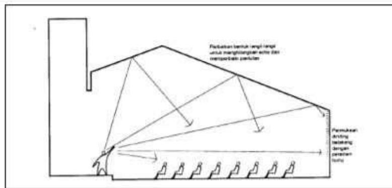
Gambar 7. Pantulan Yang Terarah Ke Audiensi
