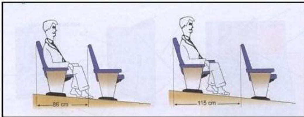
Gambar 3. Pengaturan Jarak Kursi Pada Bioskop
