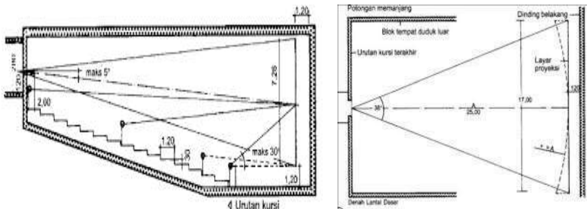
Gambar 2. Besaran Ruang Penonton Optimal
