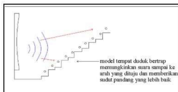
Gambar 5. Penyusunan Lantai Pada Bioskop
