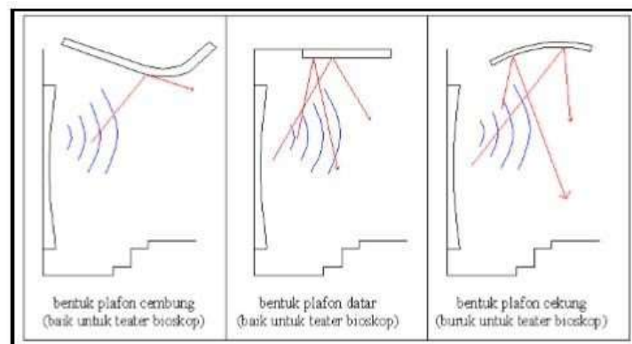
Gambar 4. Rekomendasi Bentuk Plafon Bioskop
