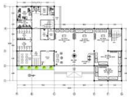
Gambar 17. Organisasi Ruang
