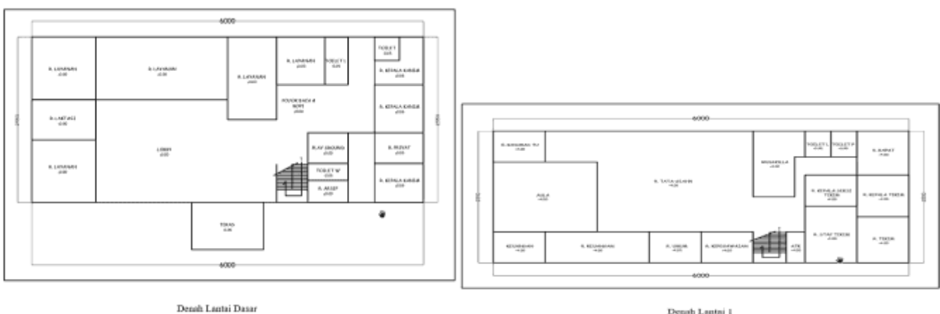
Gambar 5 Denah Eksisting Kantor Imigrasi Samarinda (Sumber: Penulis 2023)
