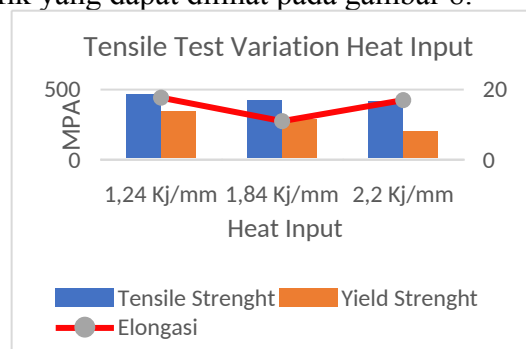
Gambar 8. Grafik Hasil Uji Tarik
