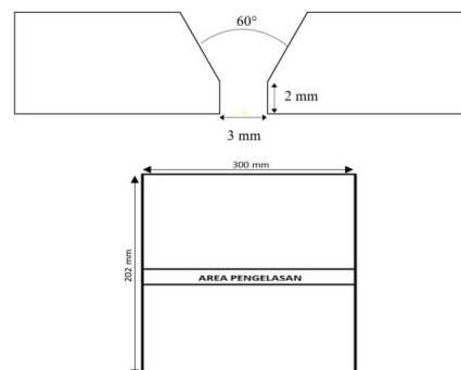
Gambar 3. Dimensi Spesimen Las
