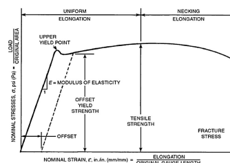
Gambar 4. Grafik Tegangan Regangan
